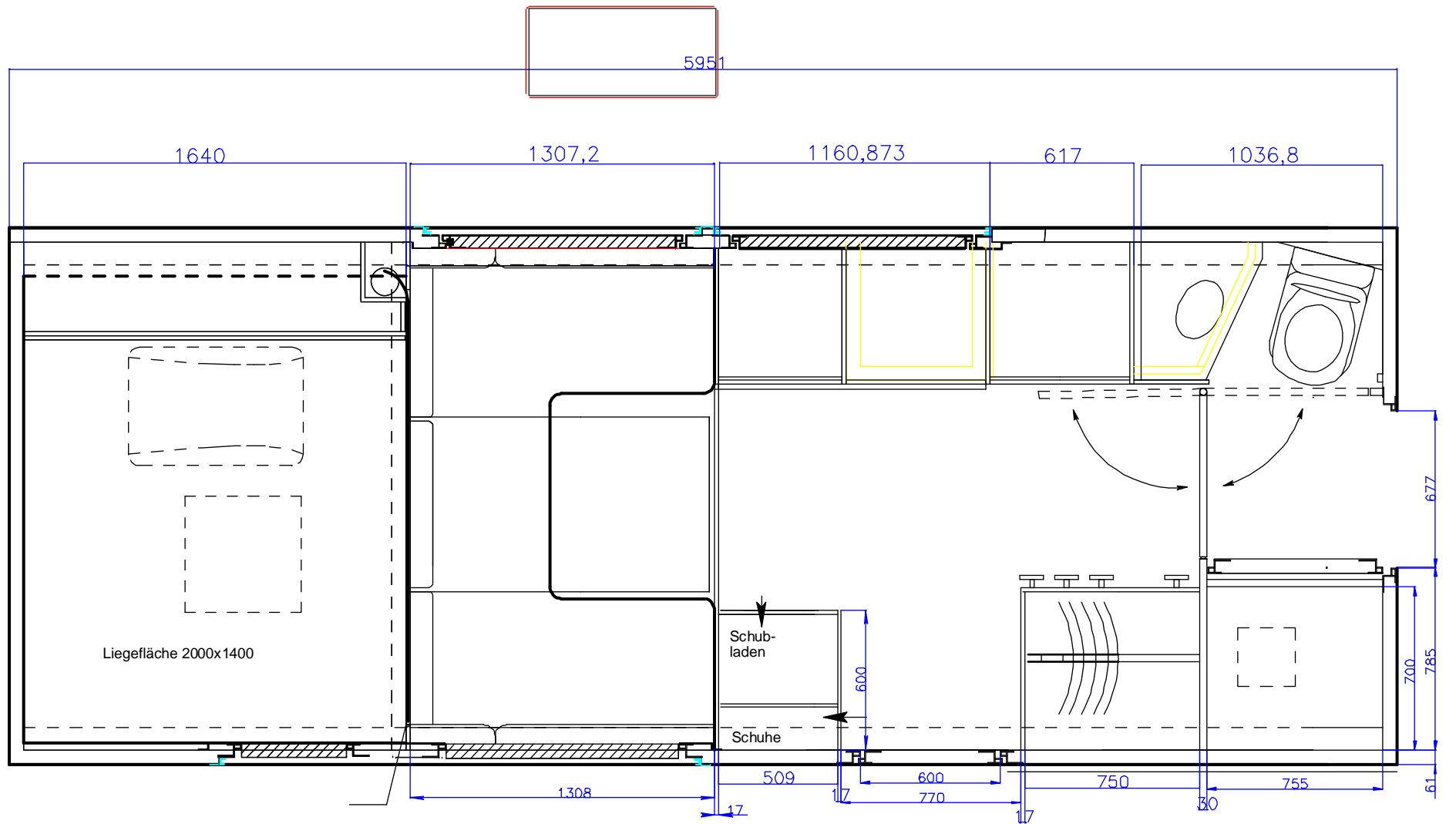
Proj. Grundriss Moebel ATACAMA L 16.9.2008 M. 1:25
